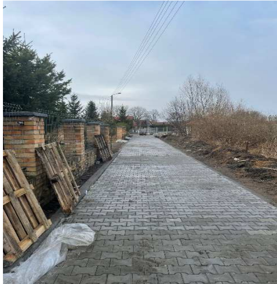
Zdjęcie 14 Budowa nawierzchni drogi w Sierakowie
